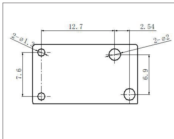
Układ wyprowadzeń PCB (widok od dołu)
