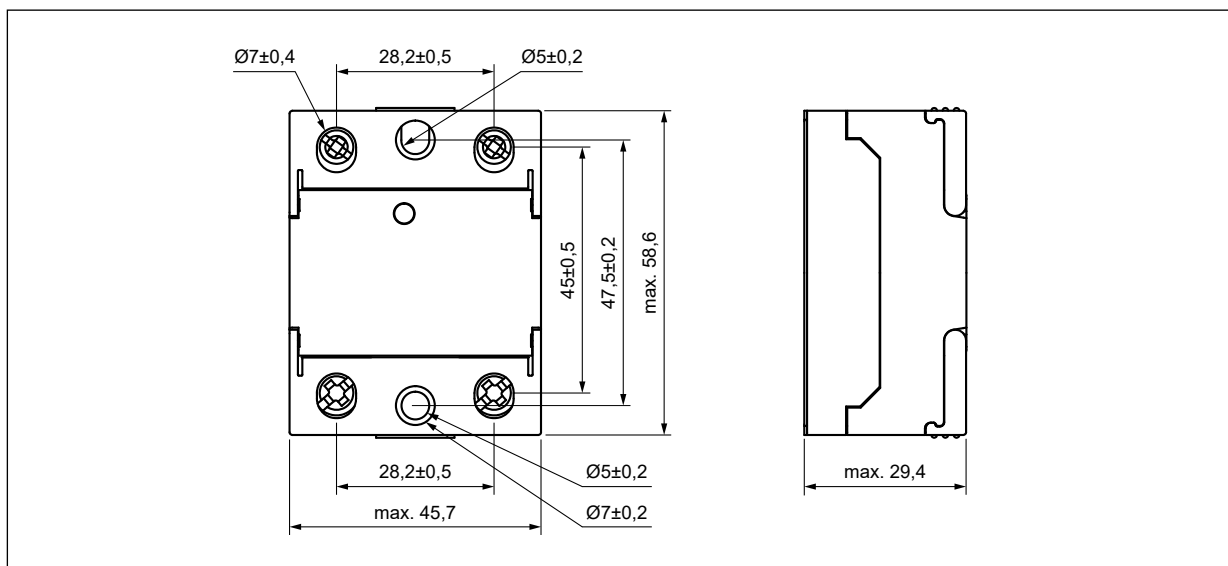
Przekaźnik półprzewodnikowy RSR54
