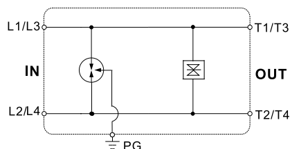
Schemat połączeń
